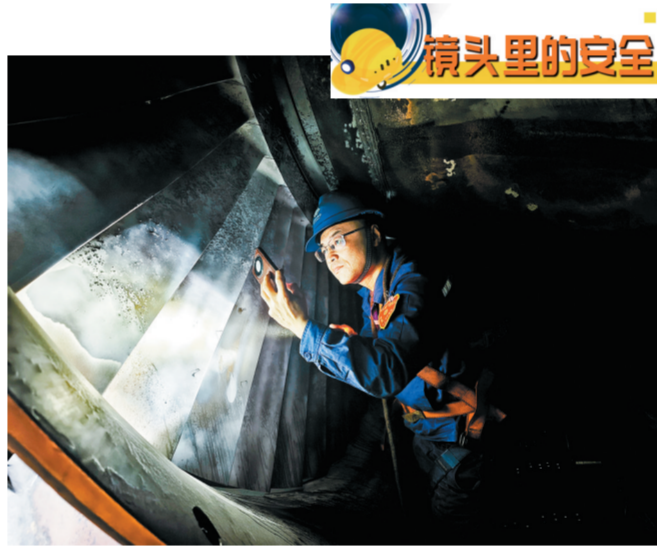
↑ 近日,山东聊城公司1号发电机转子成功抽出,检修维护人员严格按照作业指导书流程,谨遵检修工艺纪律,加紧对发电机各部位进行检查、修理。图为5月13日,技术骨干进行1号汽轮机末级叶片检查。
